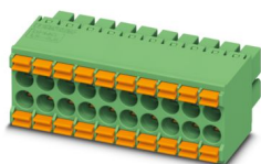
Abbildung zeigt eine 10-polige Variante mit 20 Kontakten
