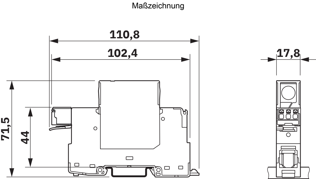
Schemazeichnung
