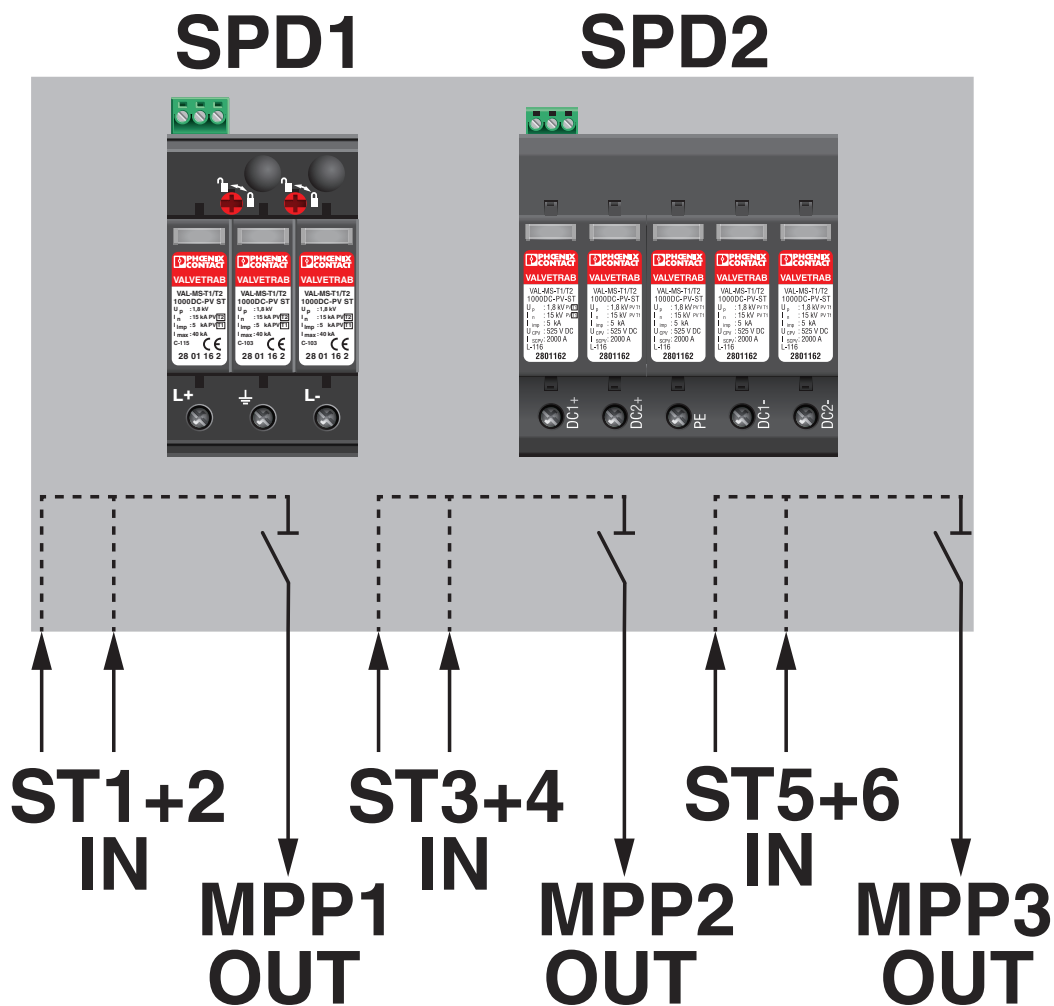
Schematische Applikationszeichnung
