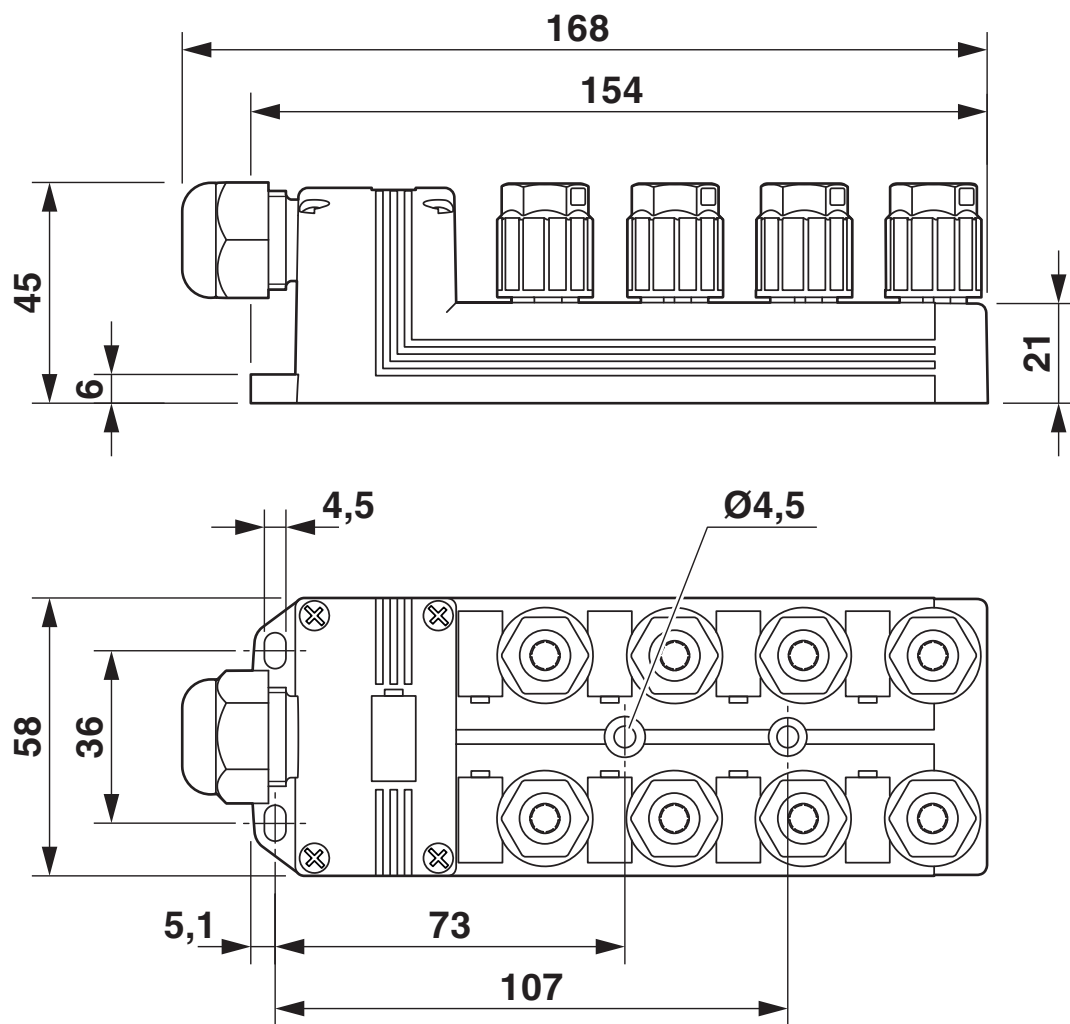
Dessin coté
