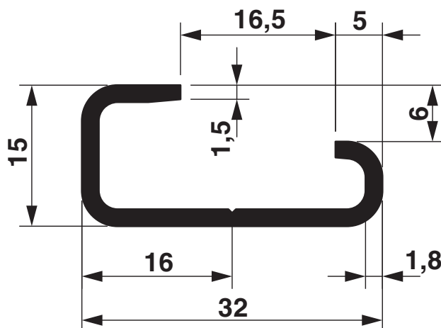
Maßzeichnung
