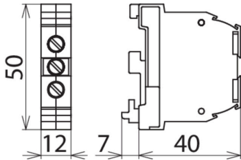
Dimensiones del SLK 16
