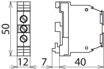
Dimensioni SLK 16
