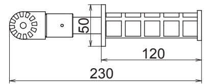
Maßbild HG ZK 230
