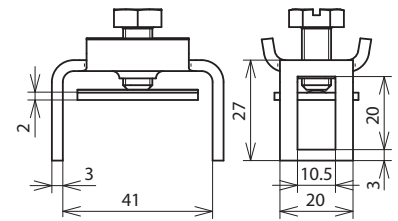
Maßbild RK FL40 PAS
