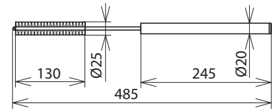
Maßbild RB 20 NS
