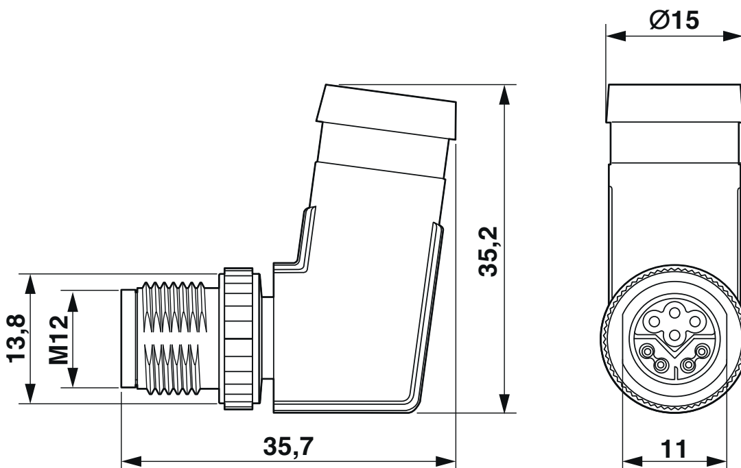
Buchse M12 x 1, gewinkelt, geschirmt
