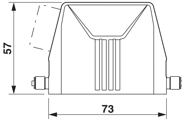
Maßzeichnung
