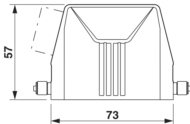
Dessin coté
