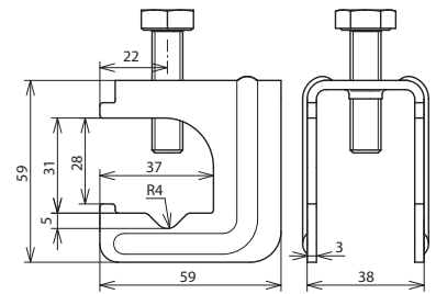
Maßbild VK 6.20 FL30 BSB STBL
