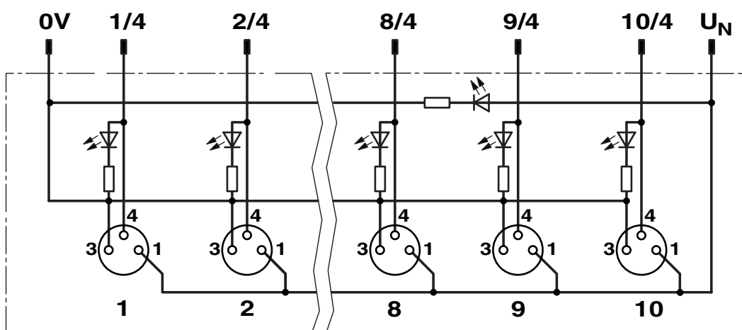
Diagrama eléctrico
