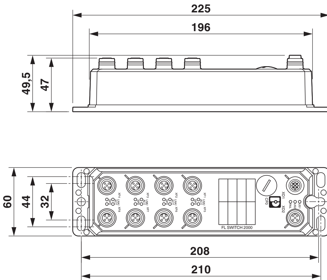
Dessin coté
