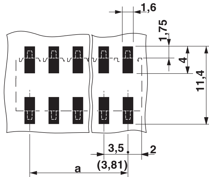
Bohrplan/Lötpadgeometrie
