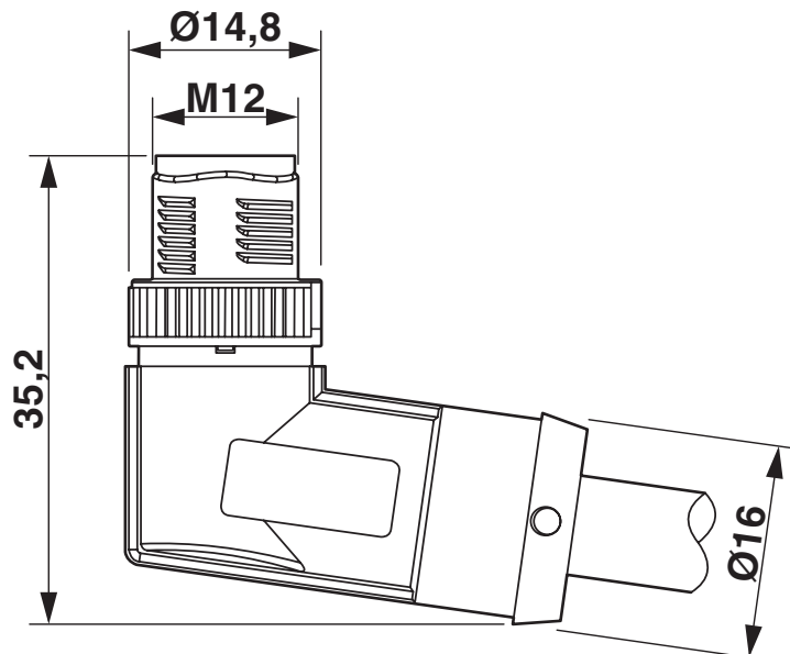
Maßzeichnung
