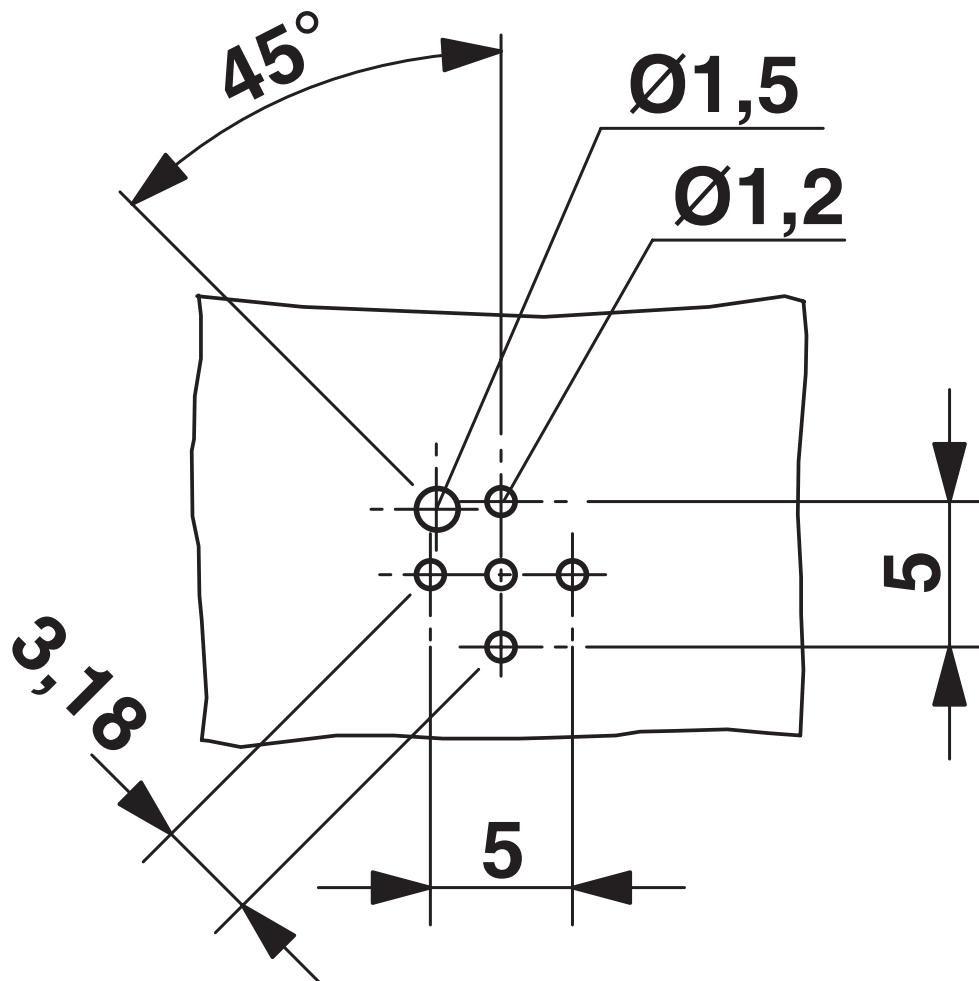
Bohrplan/Lötpadgeometrie
