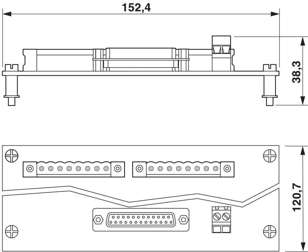
Dessin coté
