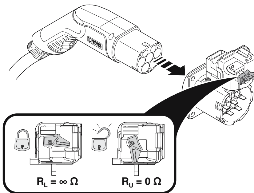
Positions du levier de déverrouillage d'urgence de l'actionneur de verrouillage
