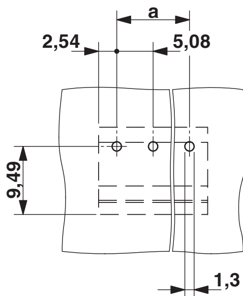
Bohrplan/Lötpadgeometrie
