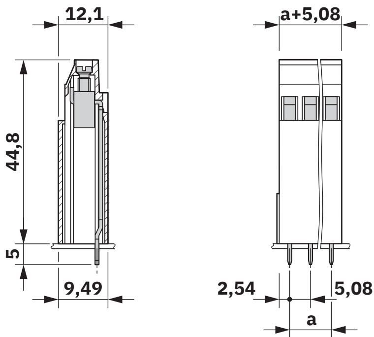
Maßzeichnung
