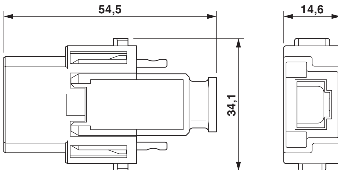
Maßzeichnung
