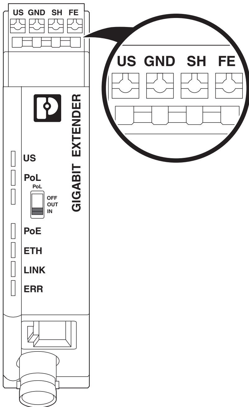
Dessin schématique
