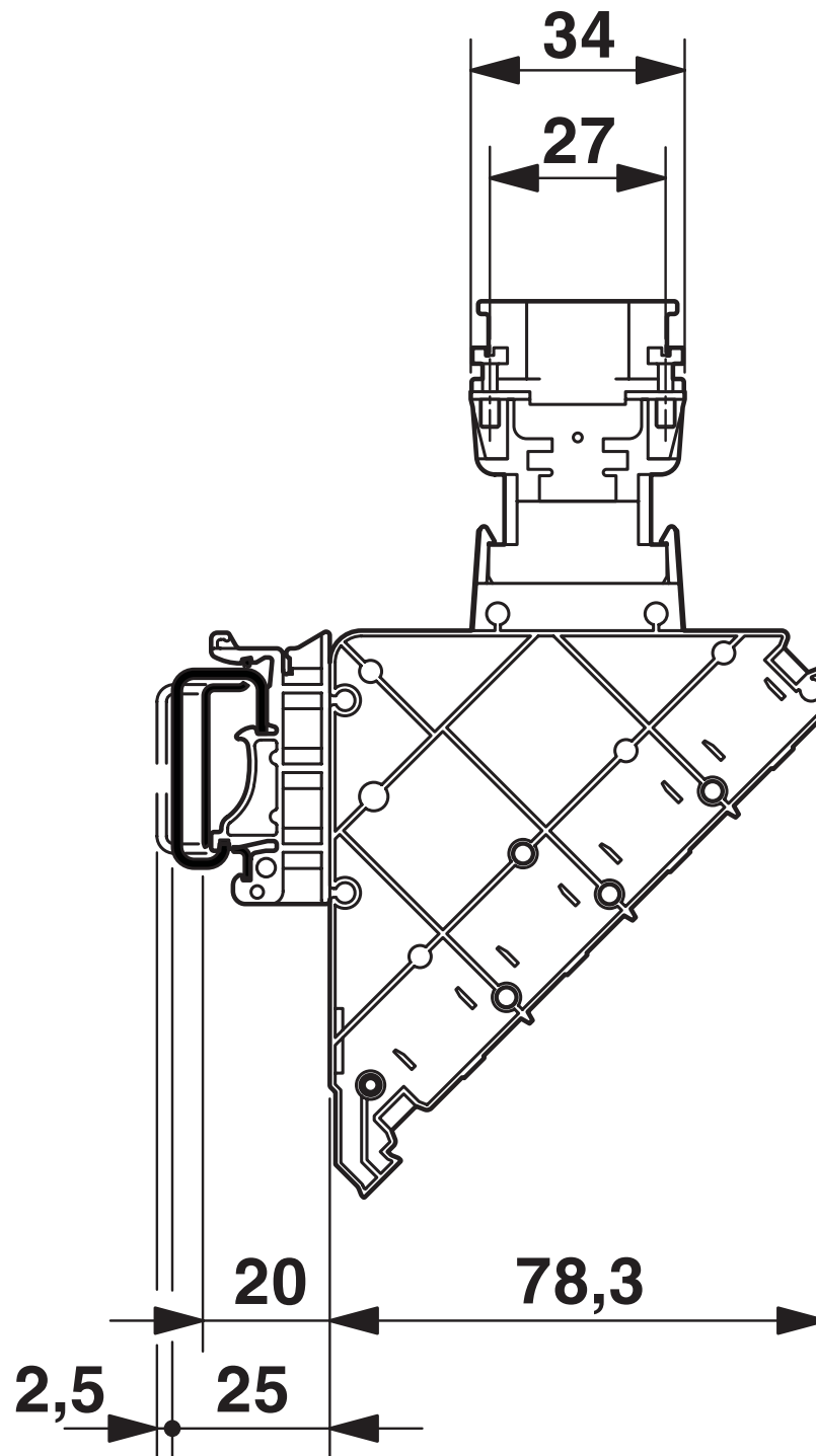
Dessin coté
