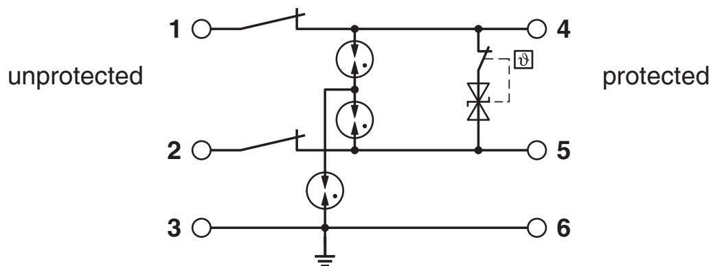
Diagrama eléctrico
