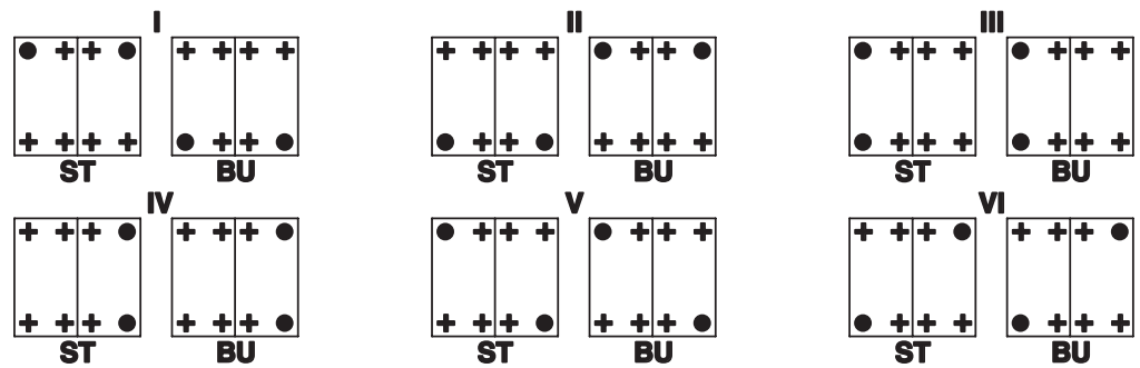
Détrompage pour capots avec deux isolants
