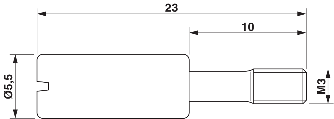
Dessin coté
