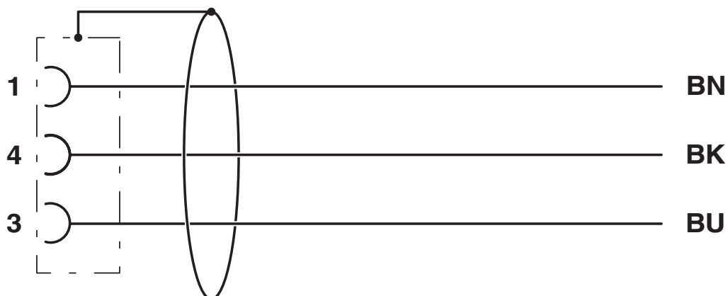
Affectation des contacts du connecteur femelle M8
