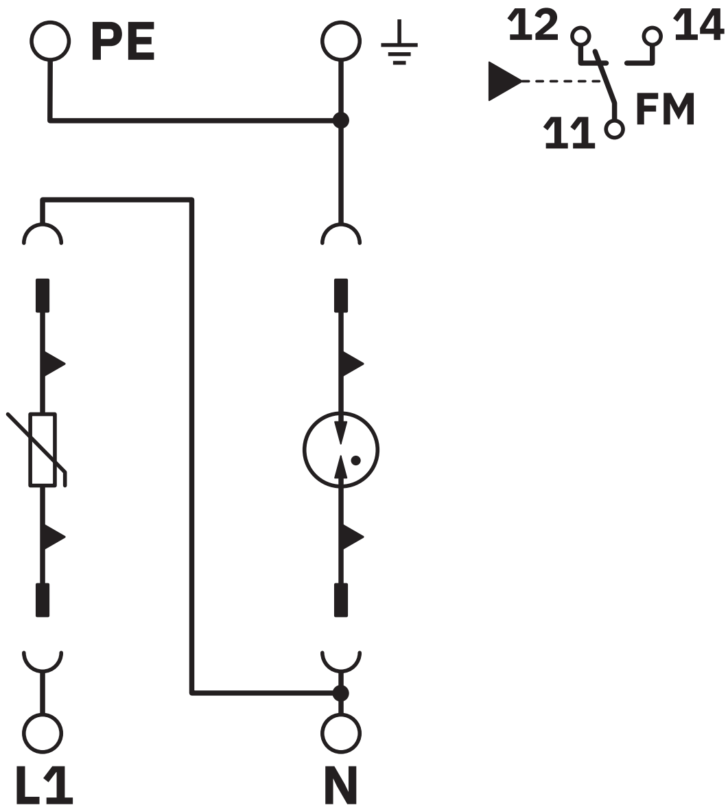
Schaltplan
