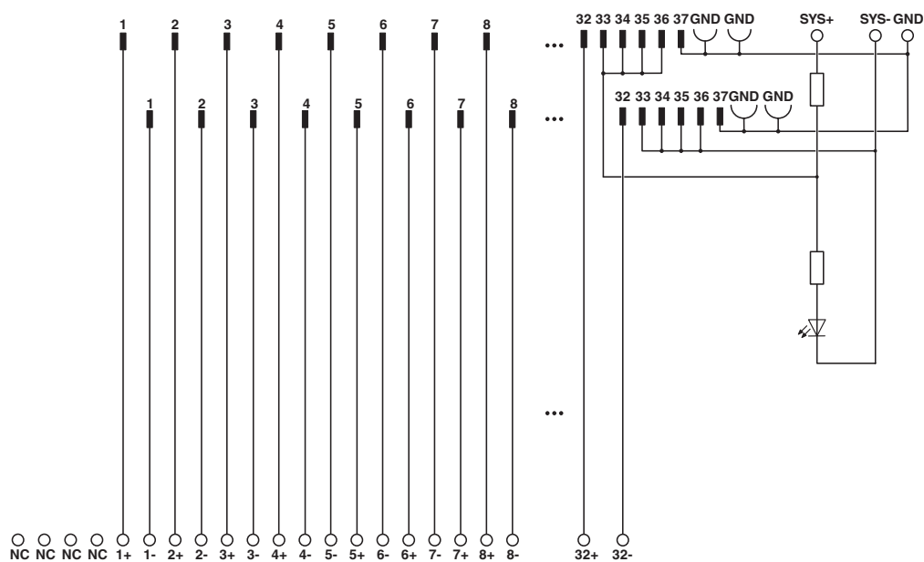
Schaltplan
