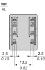
Stecker-Seitenansicht
