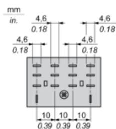
Stecker-Seitenansicht
