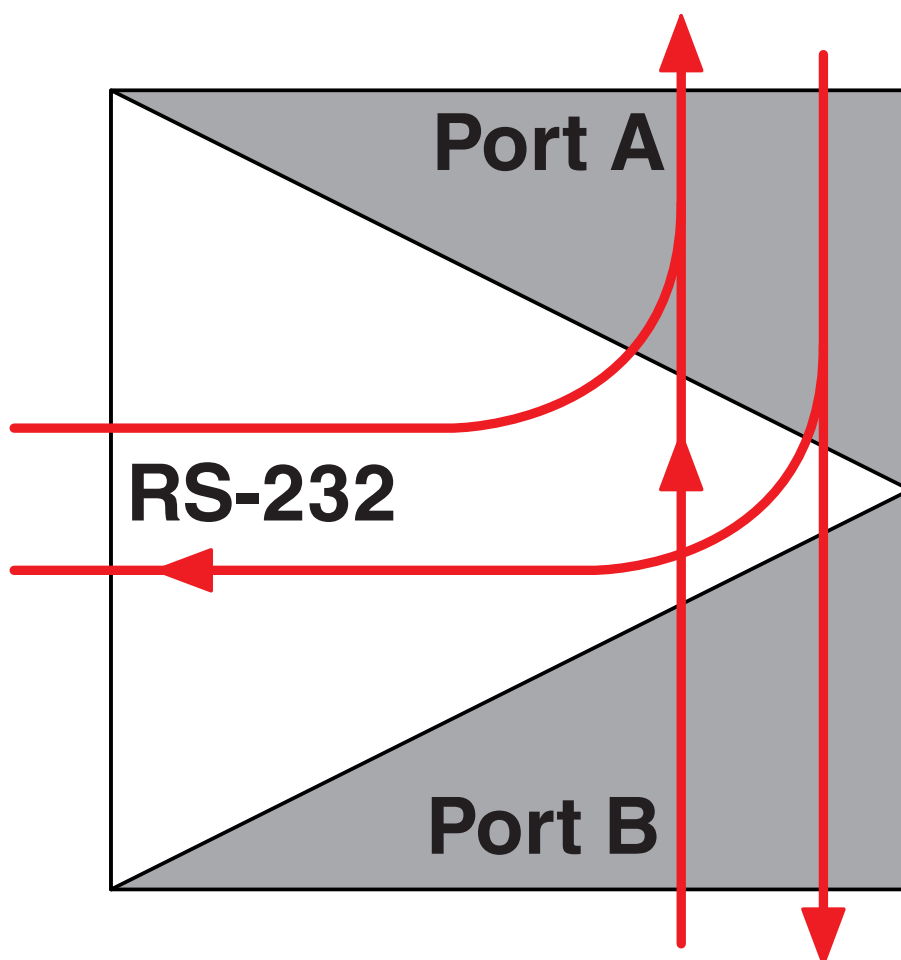
Plano esquemático
