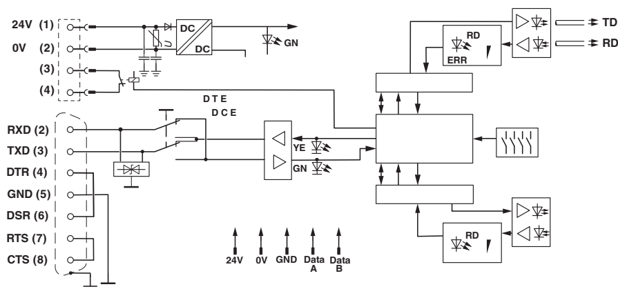
Schéma fonctionnel
