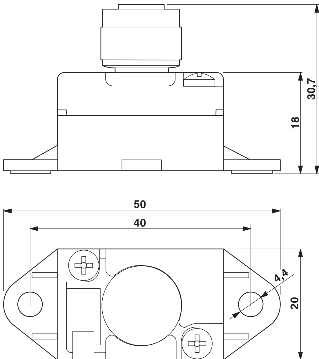
Maßzeichnung
