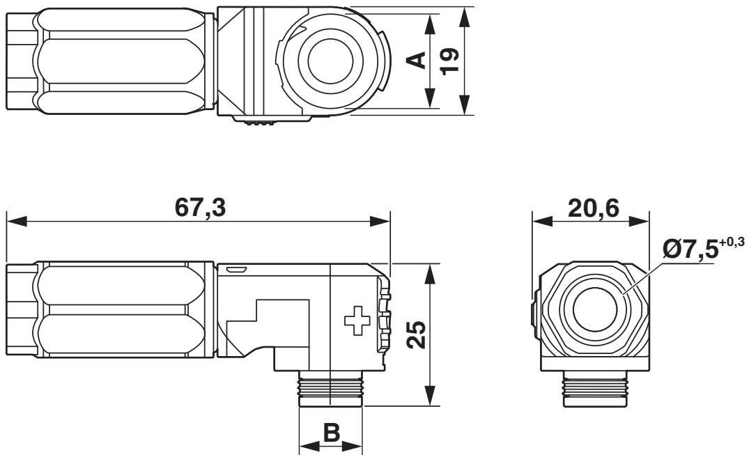
Dessin coté
