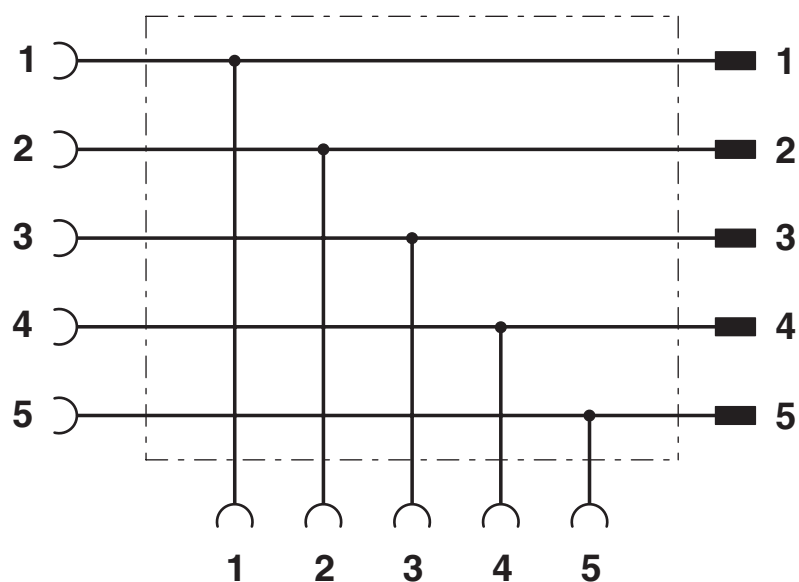
Diagrama eléctrico
