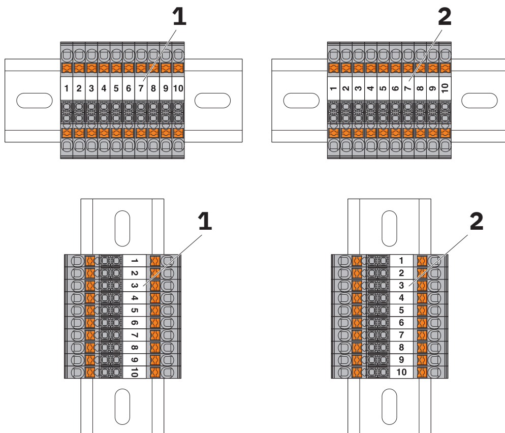
Plano esquemático
