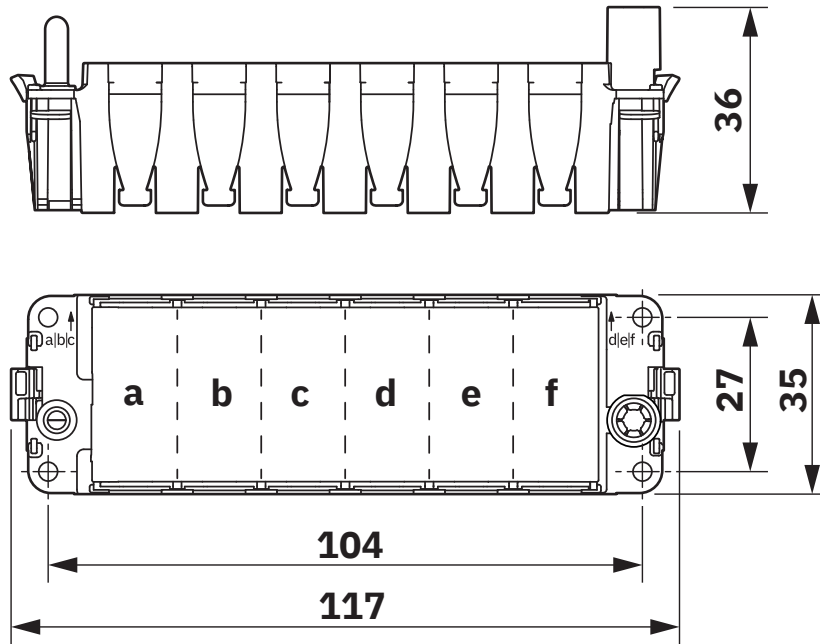
Maßzeichnung
