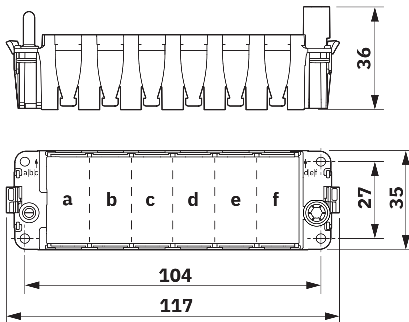
Dessin coté
