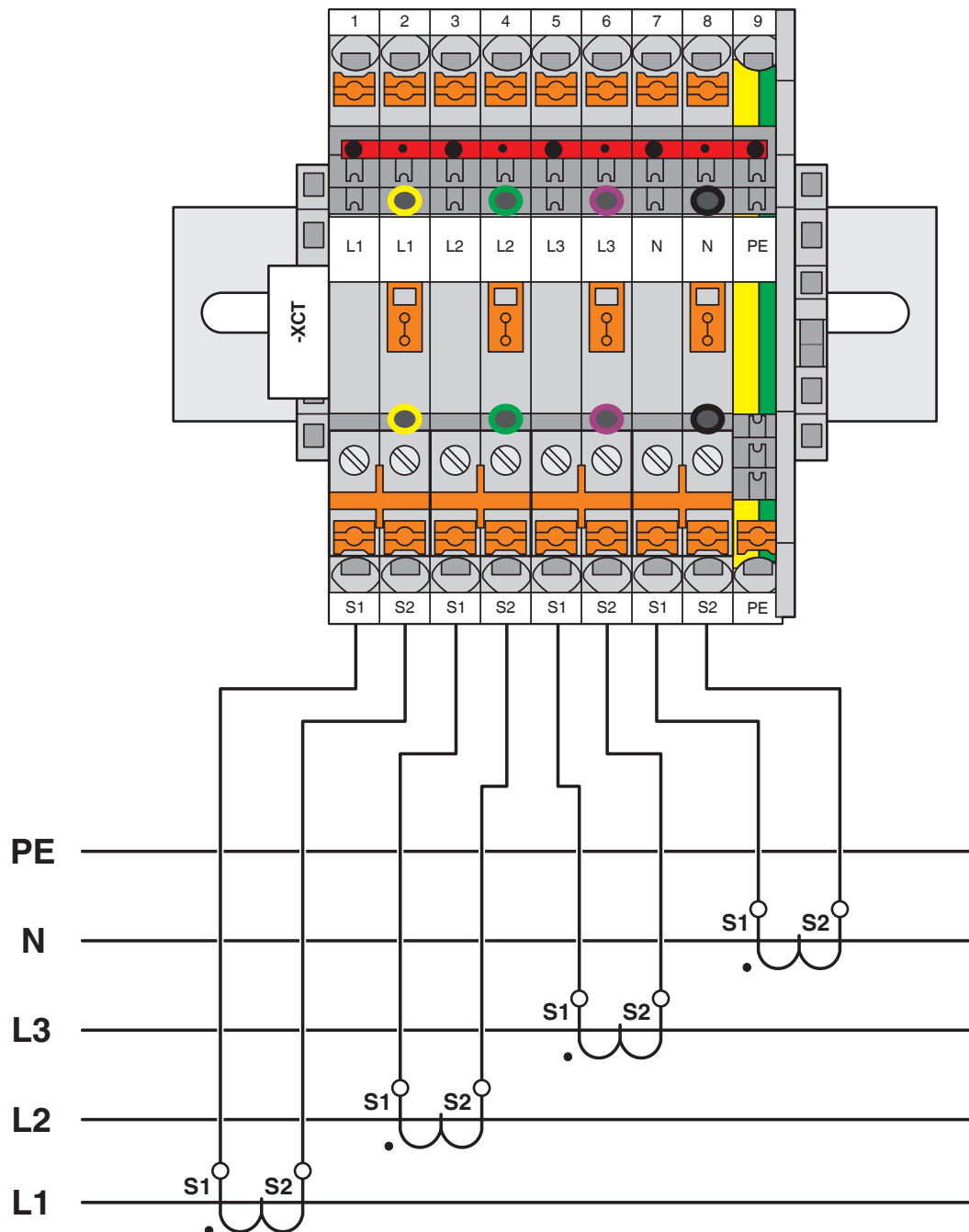
Diagrama eléctrico
