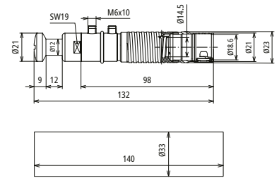
Maßbild AE ISO RIV KF HVI 60 V2A
