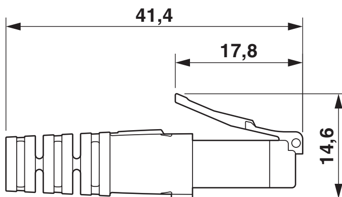
Dessin coté
