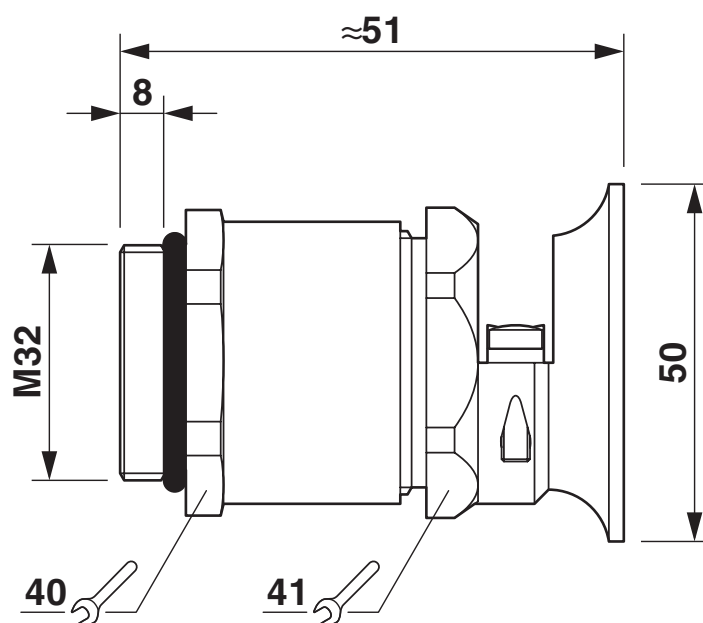
Dessin coté
