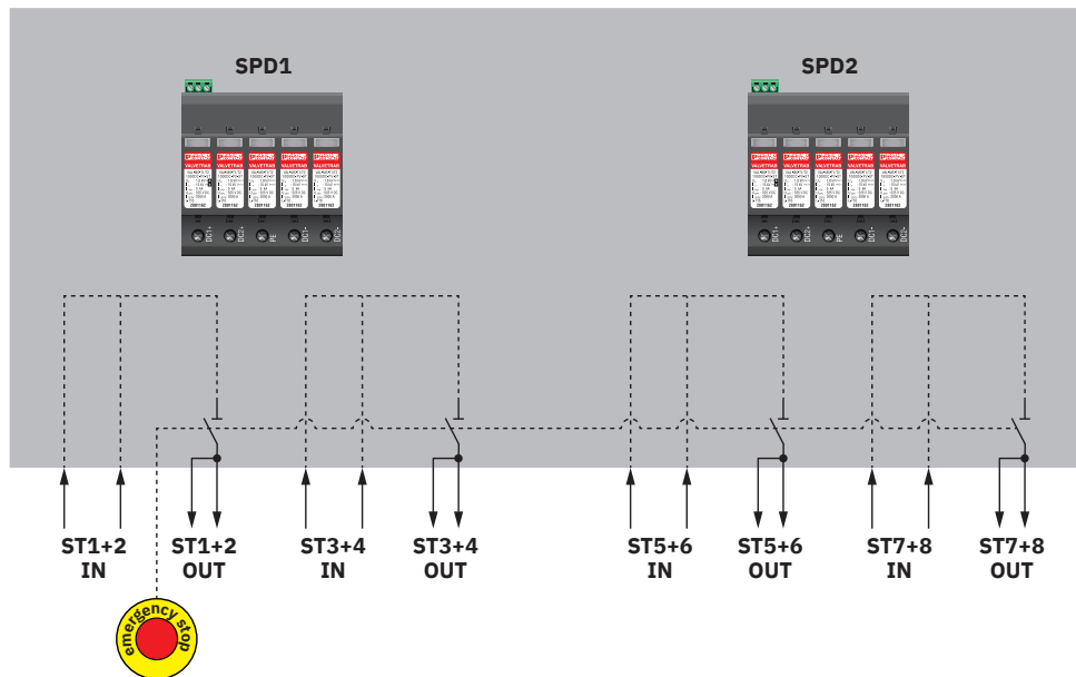
Schematische Applikationszeichnung
