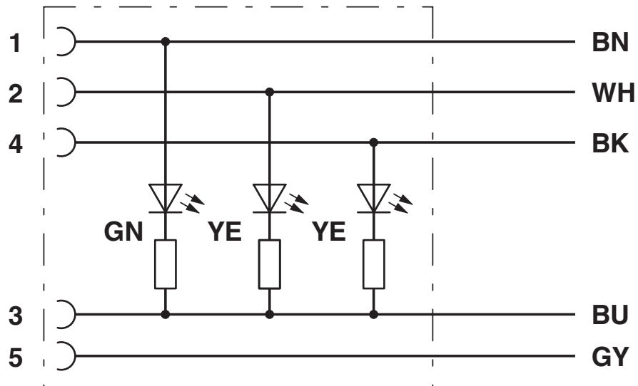
Schaltplan
