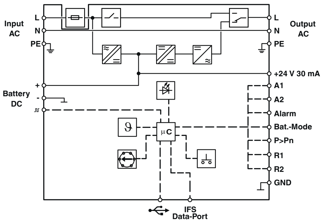
Schéma fonctionnel
