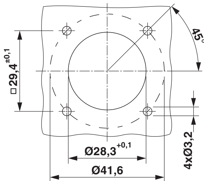
Maßzeichnung
