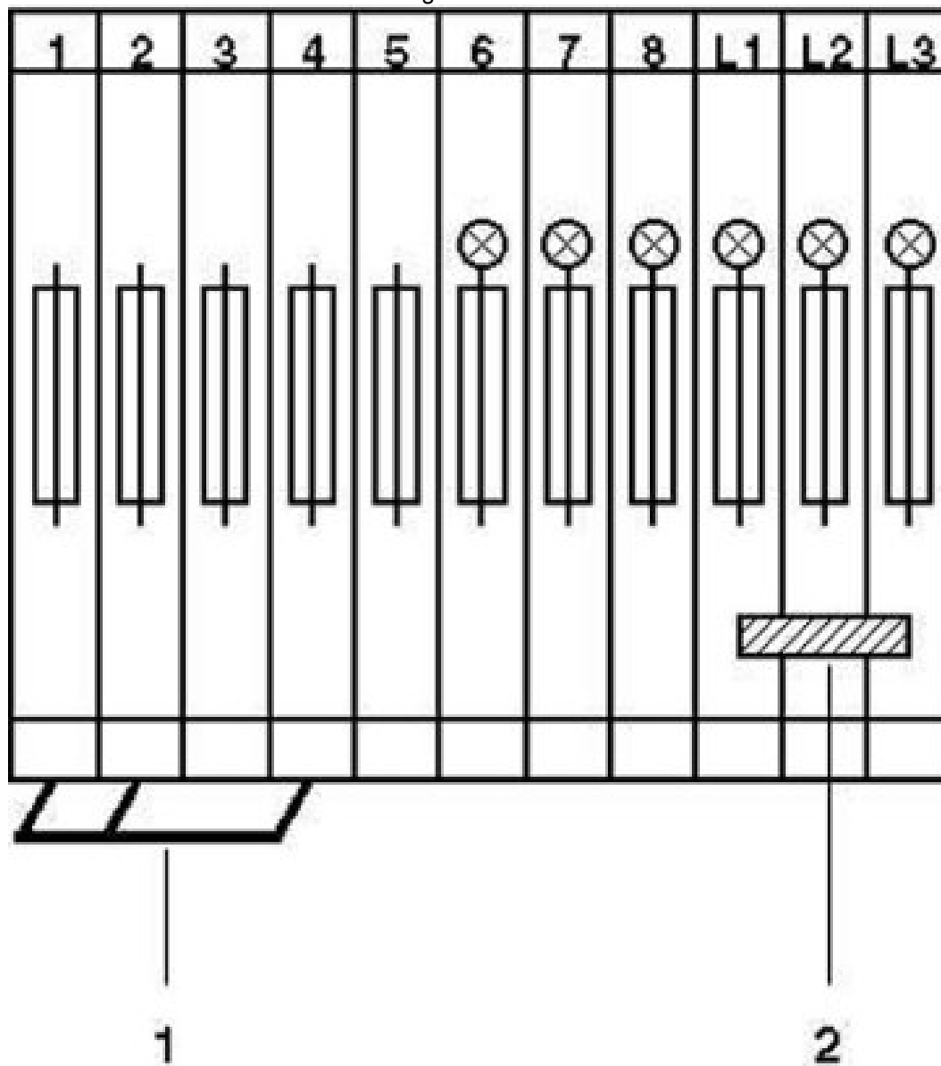
Diagrama eléctrico
