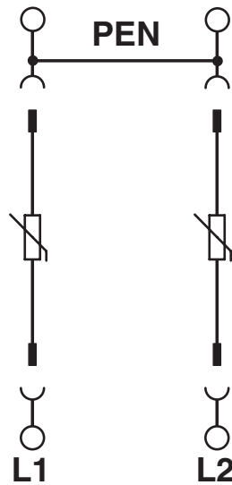
Schaltplan
